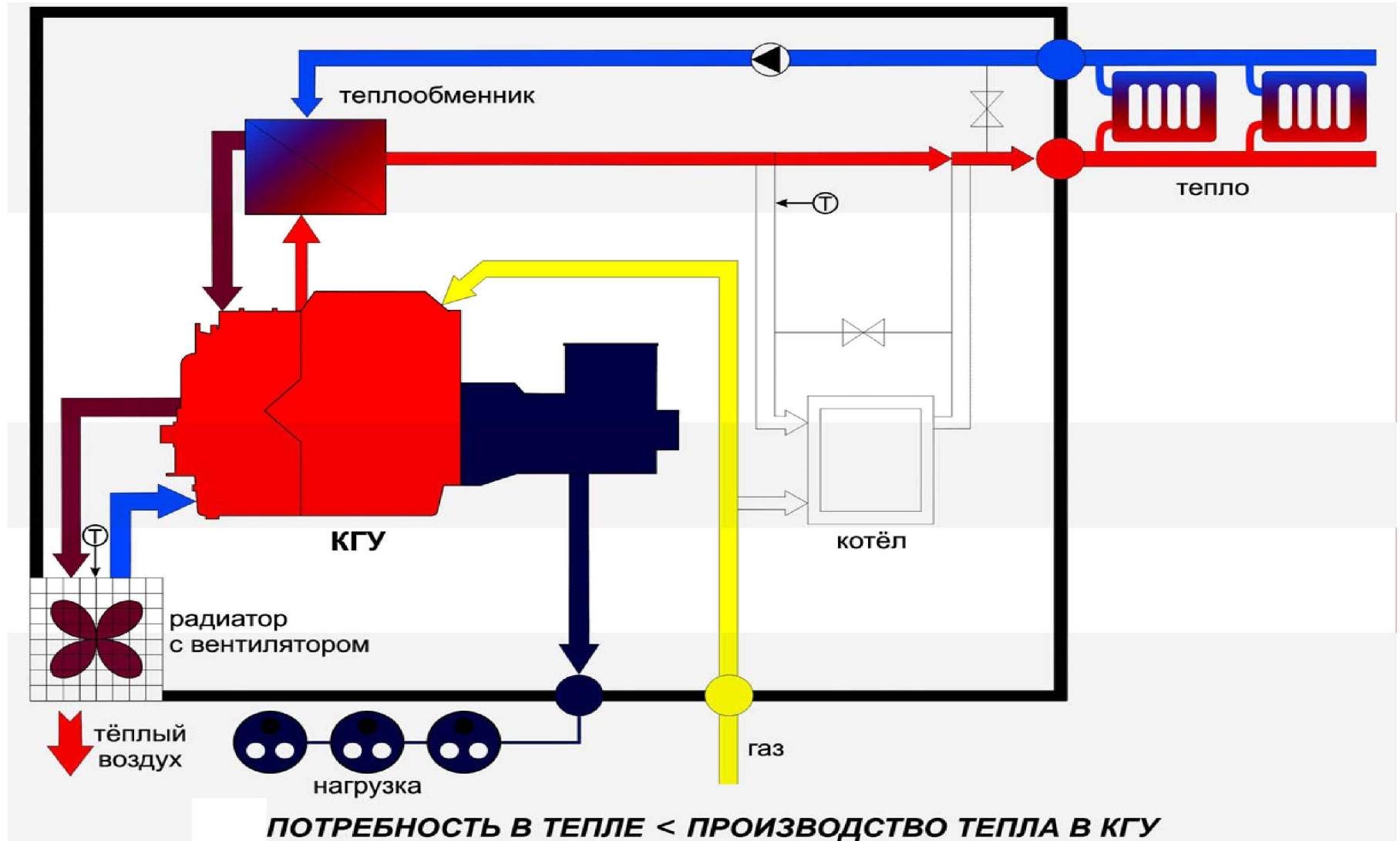
Рис. 36. Третий вариант когенераторной котельной
