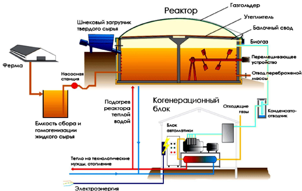
Рис. 24. Принципиальная схема биогазовой установки
