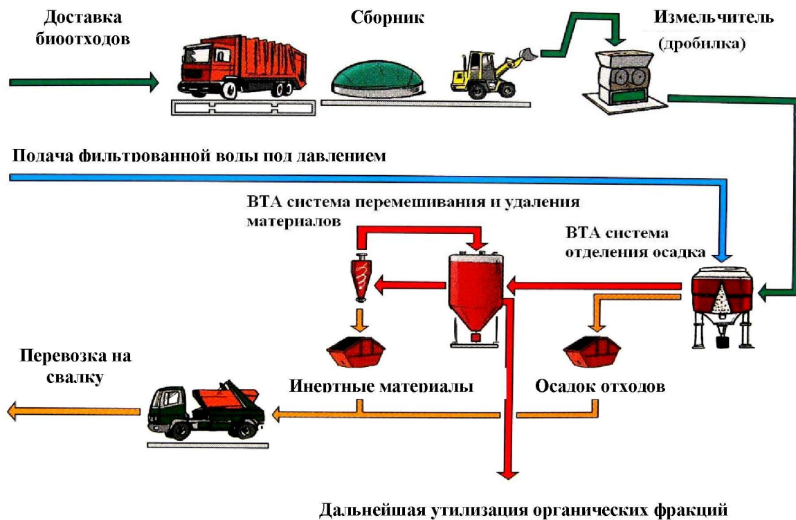
Рис. 52. Гидромеханическая система переработки отходов
