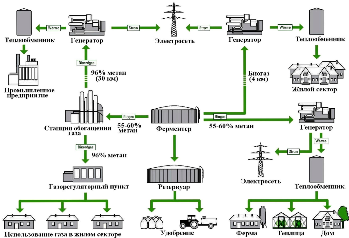
Рис. III.20. Схема использования мощной биогазовой установки (более 1000 МВт)
